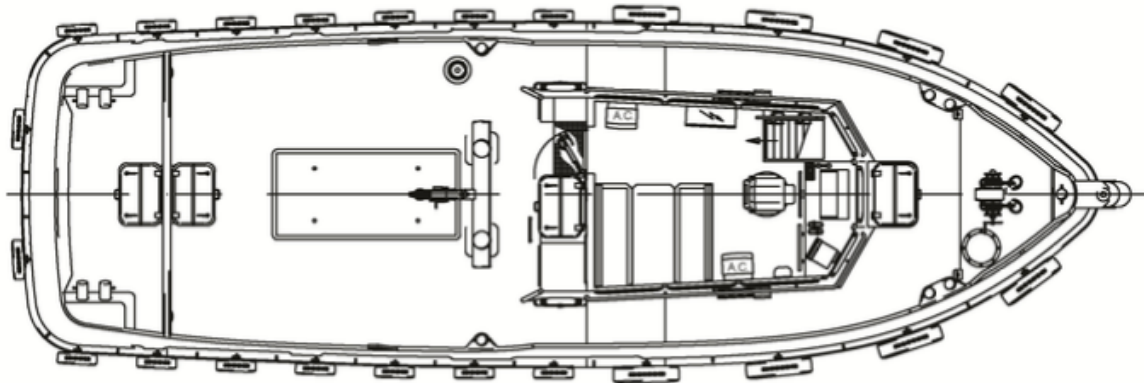
Maindeck
